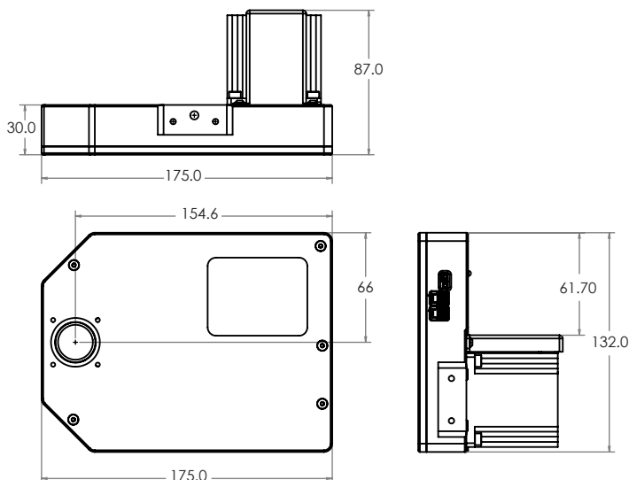
VFW1007 / VFW1010
